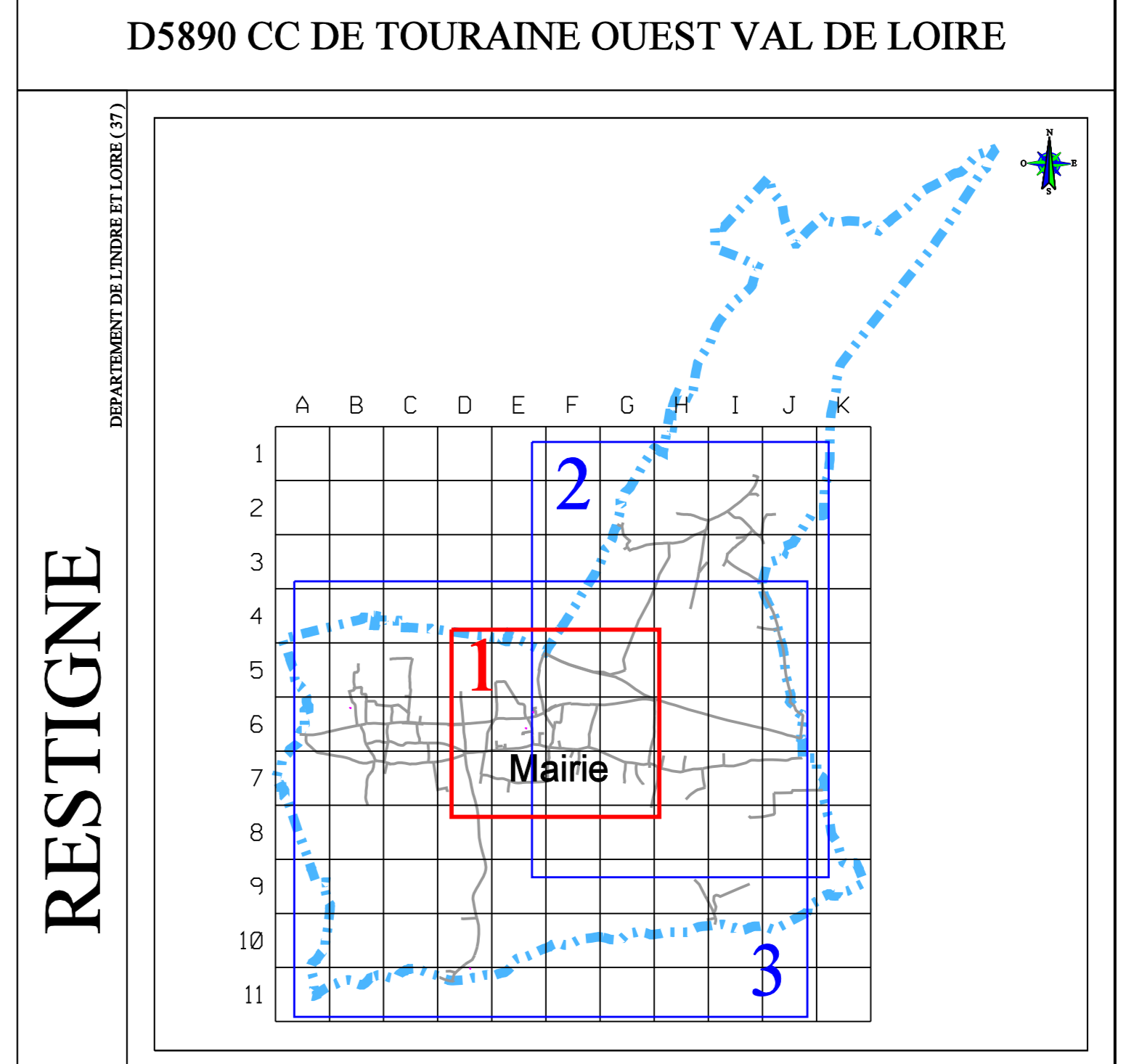
RESTIGNÉ PLAN DU RESEAU EAU POTABLE PLANCHE N° : 1 / 3
